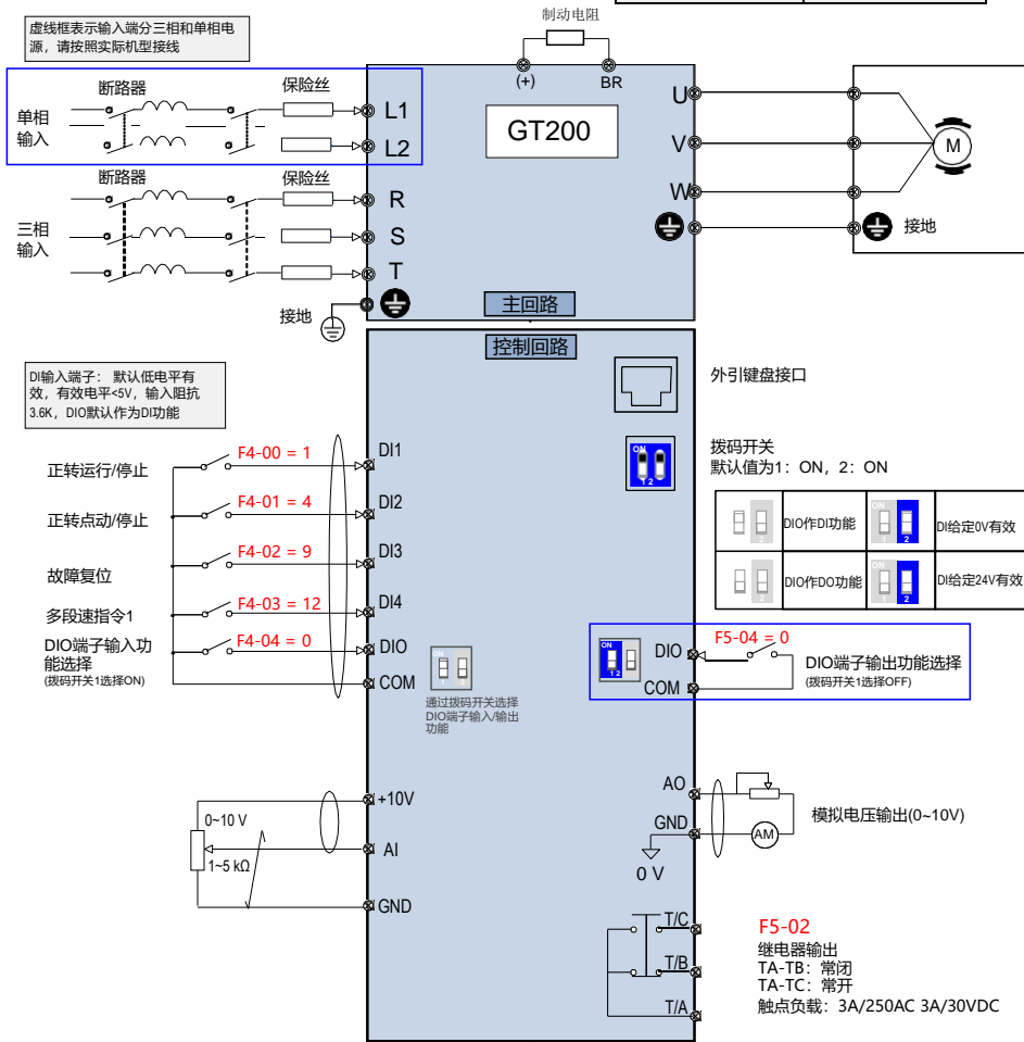
图 2-2 单相 / 三相电源输入 (GT200-2S0.4B-NC~GT200-2S2.2B-NC, GT200-4T0.4B-NC~GT200-4T3.7B-NC) 端子接线图
