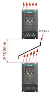
上下安装
