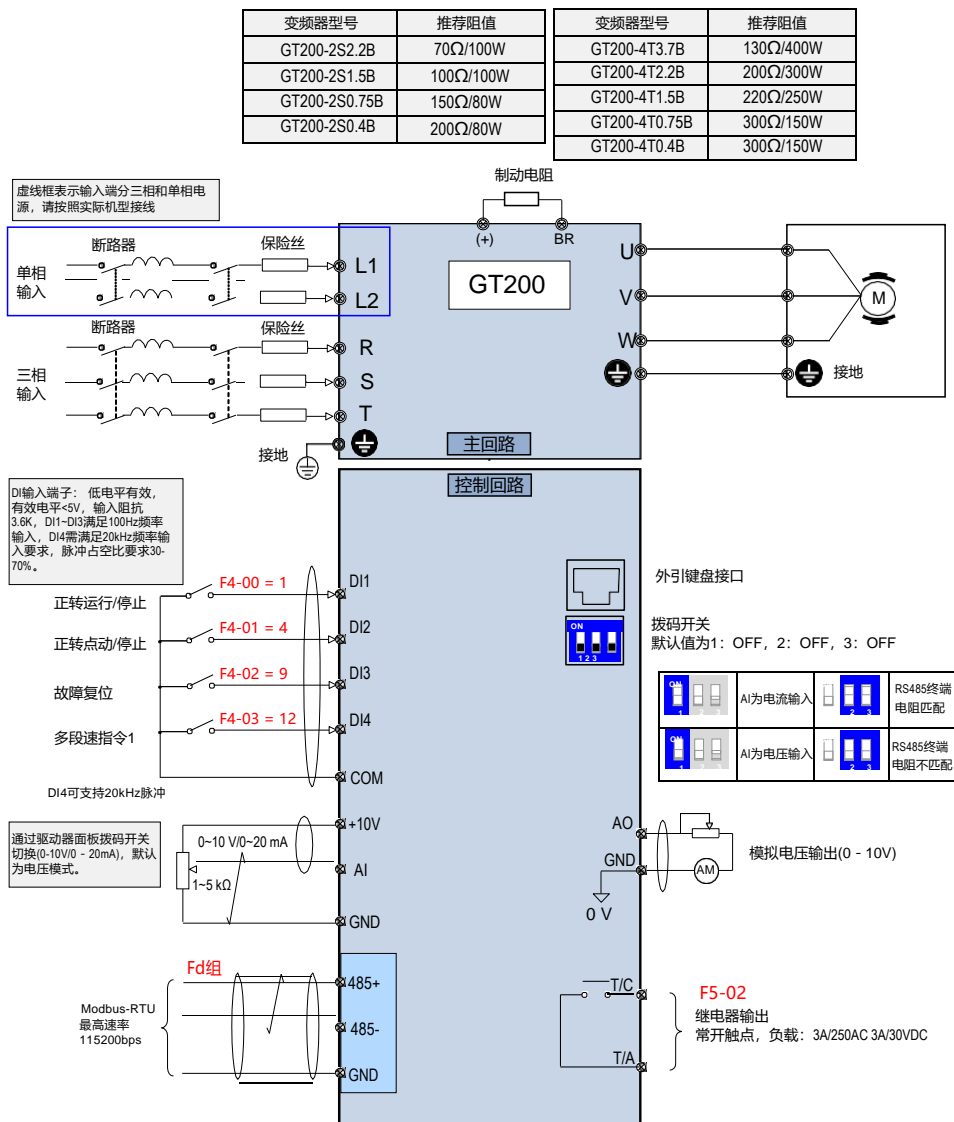
图 2-1 单相 / 三相电源输入 (GT200-2S0.4B~GT200-2S2.2B, GT200-4T0.4B~GT200-4T3.7B) 端子接线图
