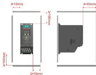
单机安装
